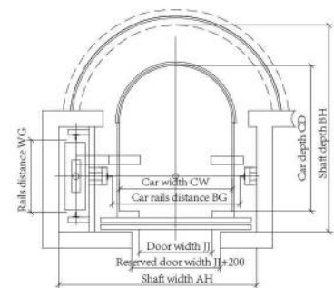
Shaft layout(Semi-circular)
