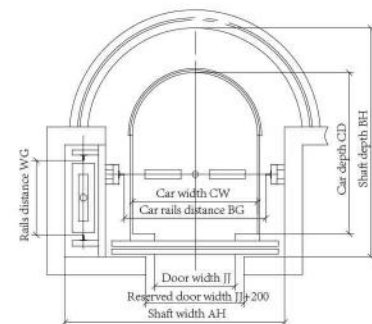
Shaft layout(Semi-circular)
