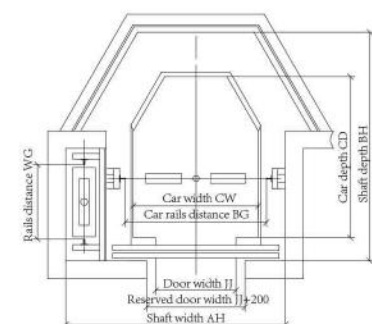
Shaft layout(diamond)
