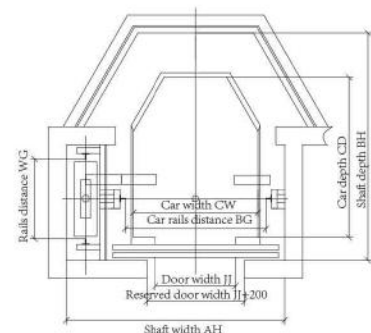
Shaft layout(diamond)
